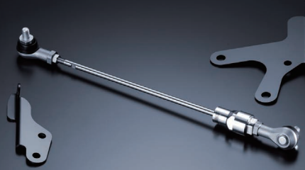
■STI フレキシブルドロースティフナー フロント◆ ¥34,760 [¥28,000+税¥3,600] ST20118VR000 ●クロスメンバーとロアアーム右側締結部の間に装着。
