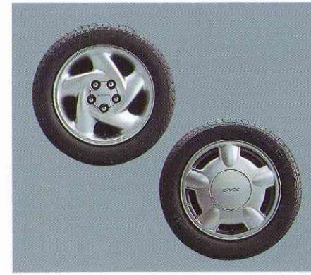
⑥225/50R16 92Vラジアルタイヤ(ボテンザRE71) & アルミホイール(タービンタイプ(上)、ディッシュタイプ(下)も選択可能)
