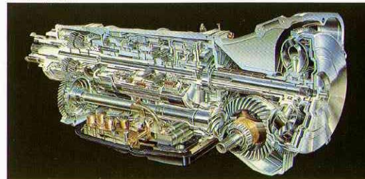
E-4AT断面図
