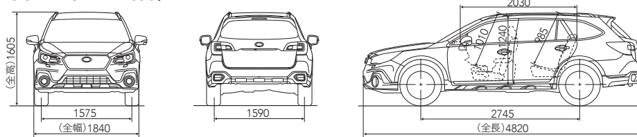
3面図(LEGACY OUTBACK Limited) 単位: mm
