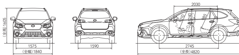
3面図(LEGACY OUTBACK Limited) 単位：mm
