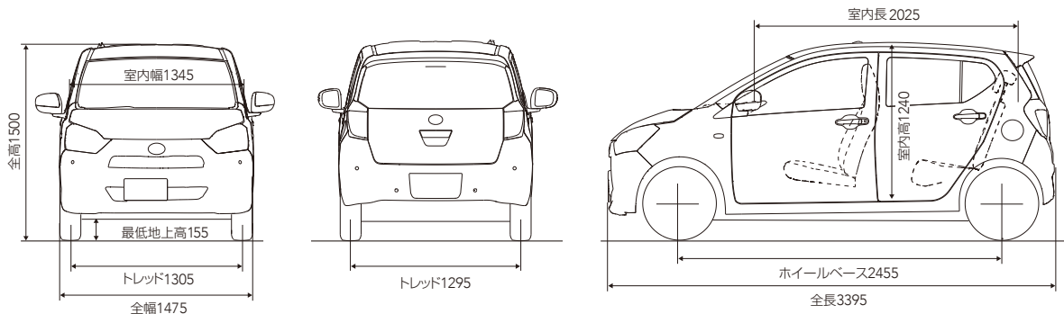
3面図 (G 2WD車) 単位: mm
