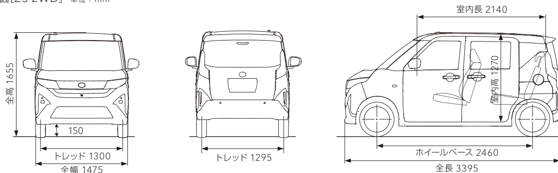
3面図[ZS 2WD] 単位: mm
